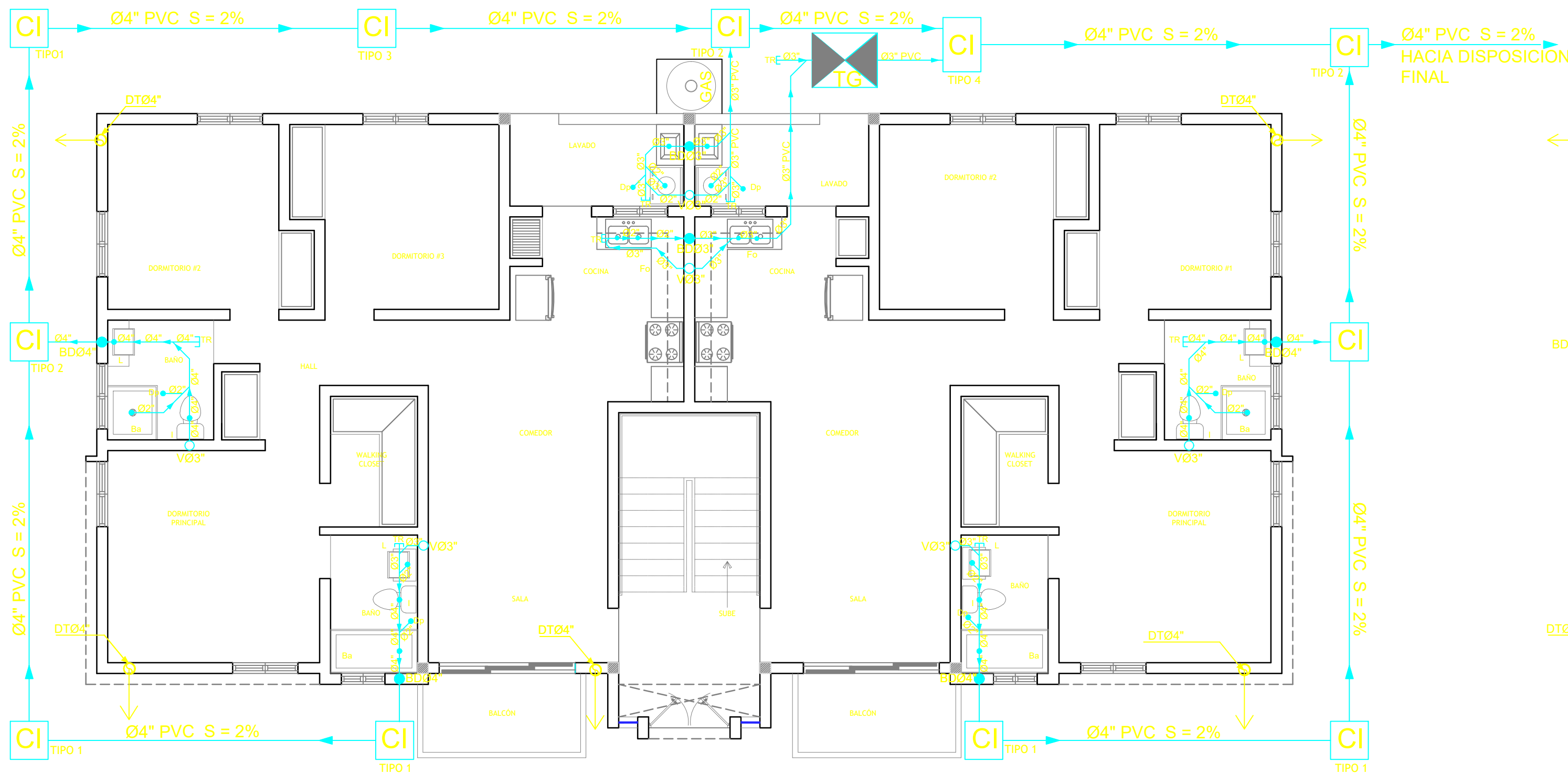
PLANTA RECOLECCION AGUAS RESIDUALES DE 1ER. NIVEL, BLOQUE B ESCALA: 1:75
