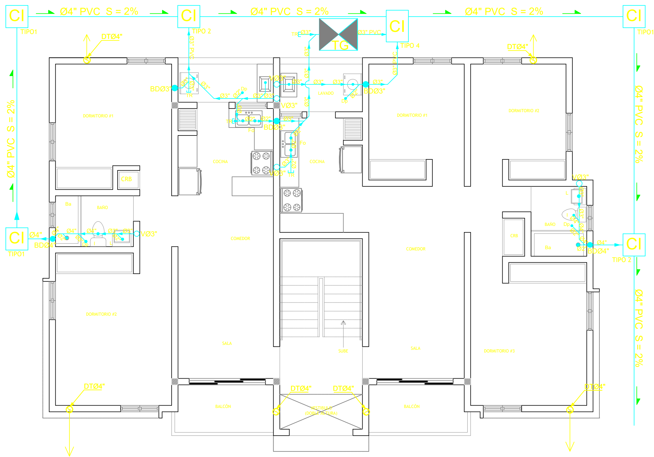
PLANTA RECOLECCION AGUAS RESIDUALES DE 1ER. NIVEL, BLOQUE A ESCALA: 1:75
