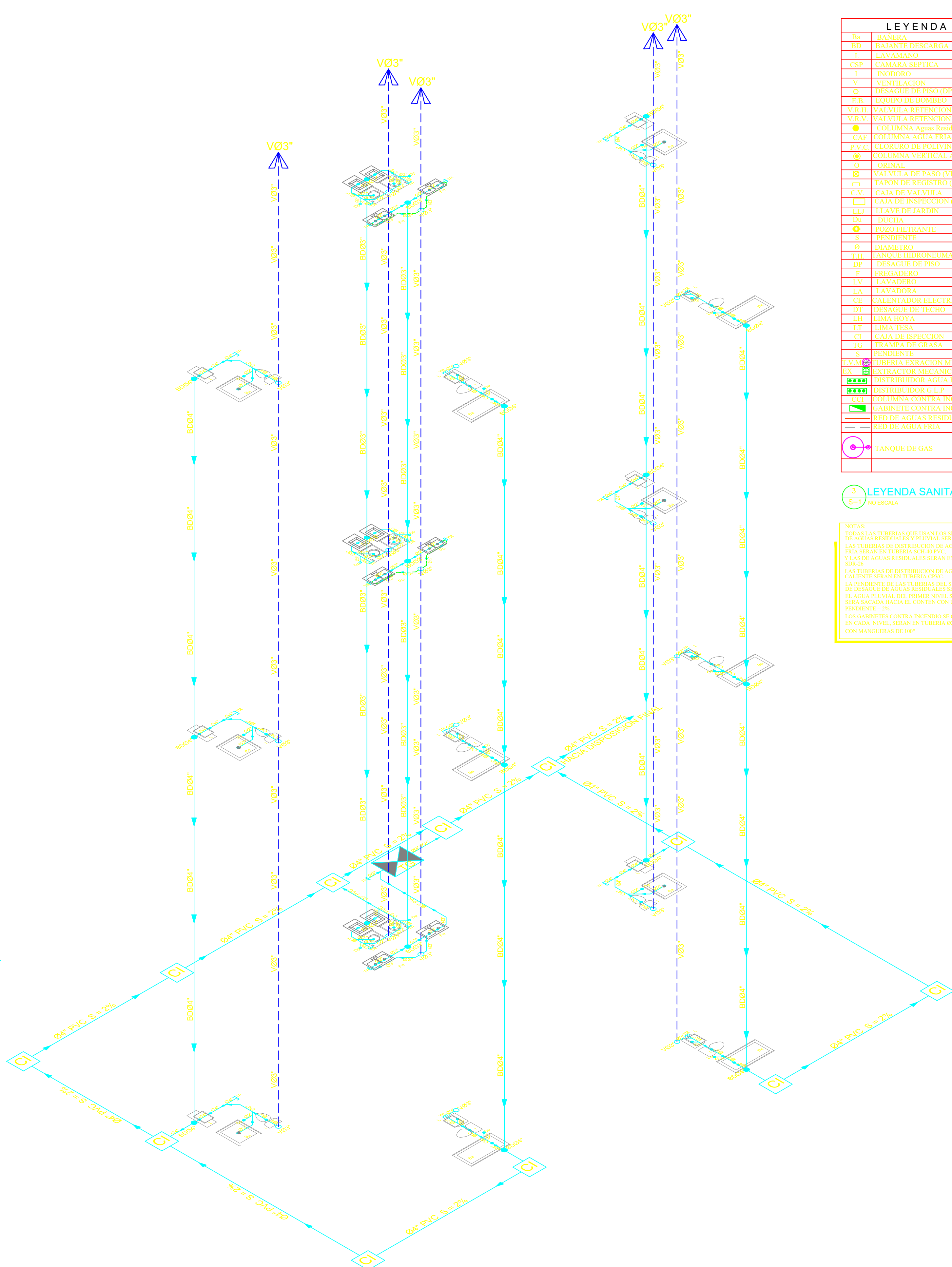
PERSPECTIVA ISOMETRICA AGUAS RESIDUALES BLOQUE A NO ESCALA
