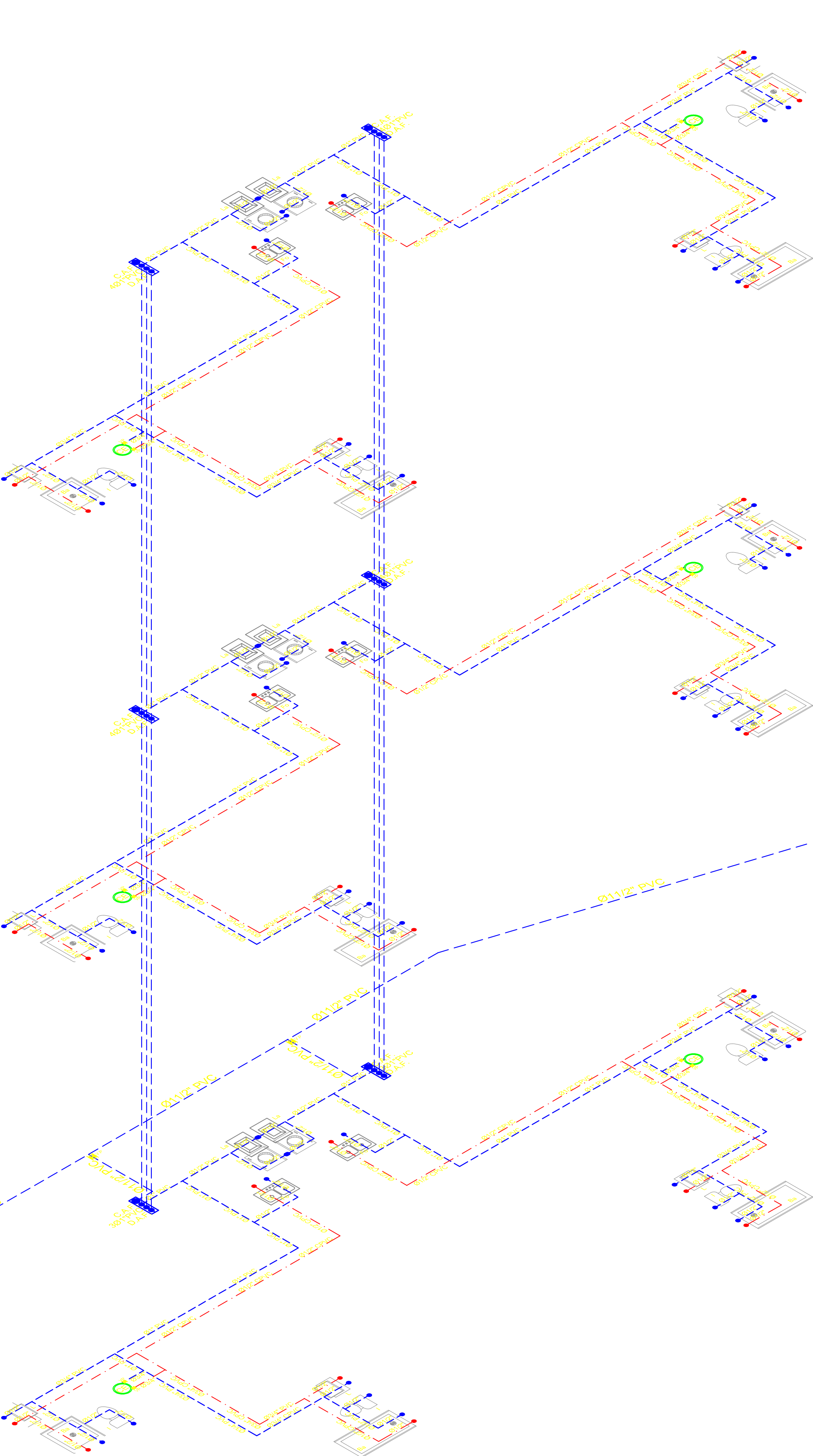
PERSPECTIVA ISOMETRICA AGUA FRIA Y CALIENTE BLOQUE A NO ESCALA
