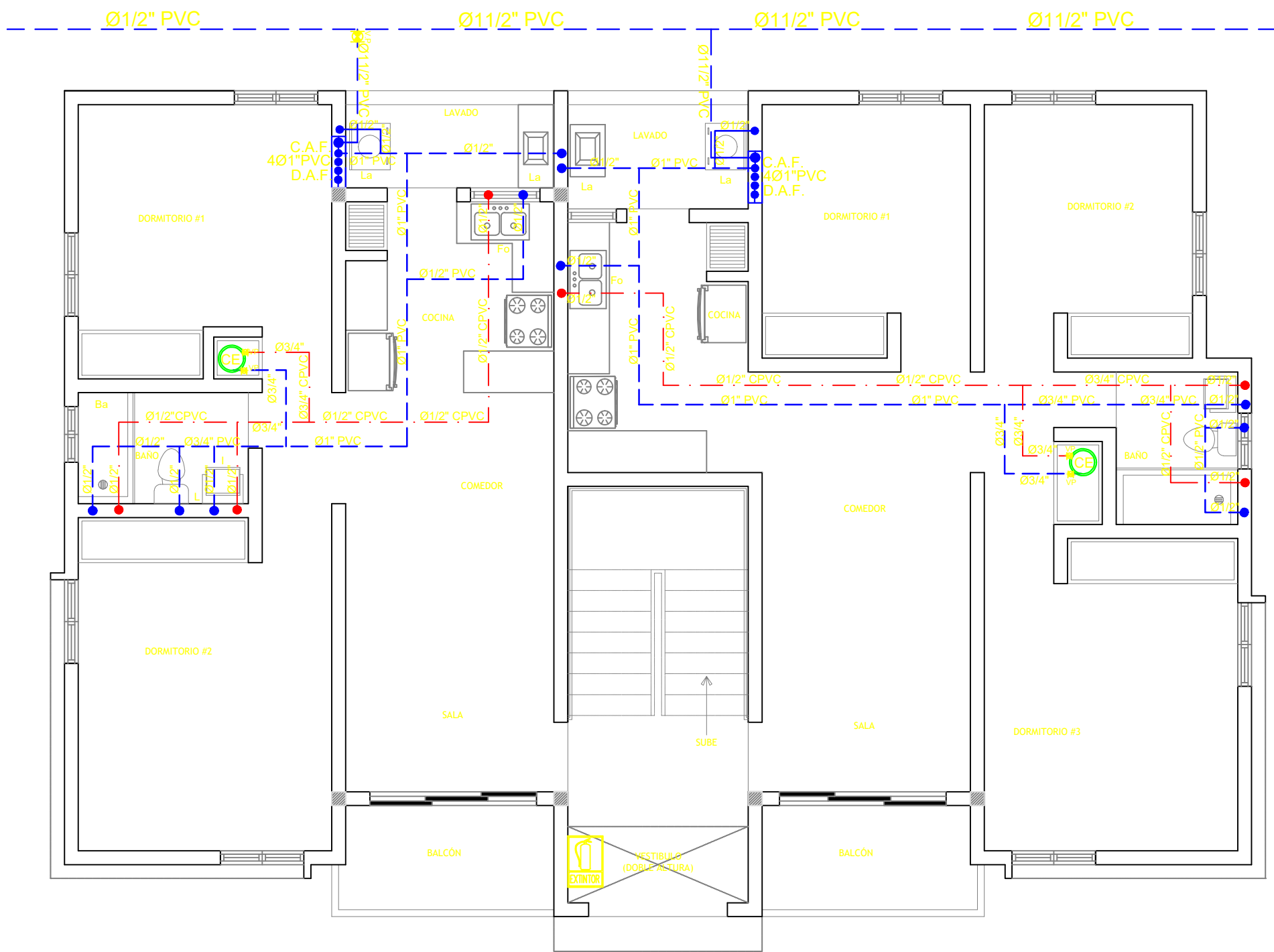
PLANTA DISTRIBUCION AGUA FRIA Y CALIENTE DE 1ER. NIVEL, BLOQUE A ESCALA: 1:75
