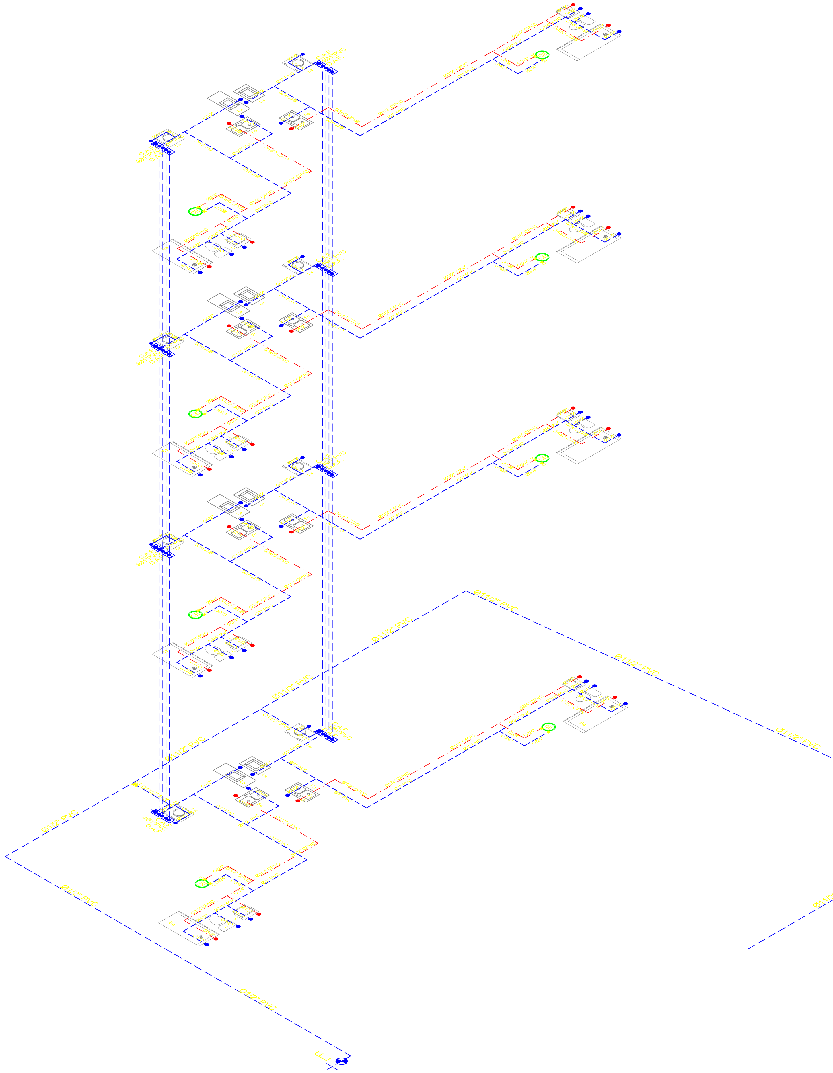
PERSPECTIVA ISOMETRICA AGUA FRIA Y CALIENTE BLOQUE B NO ESCALA
