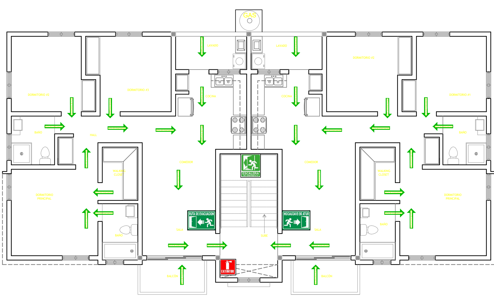
PLANTA RUTA EVACUACION 2DO. AL 3ER NIVEL, BLOQUE B ESCALA: 1:75
